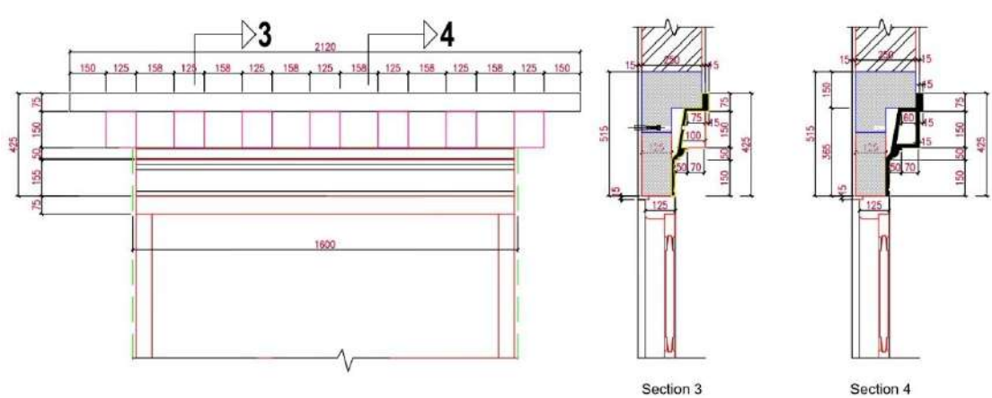
Fig 5.11.4 GRC Door Cornice 1410mm dhung length
